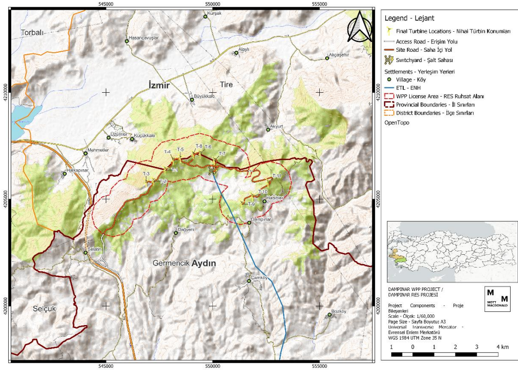
Figür 1.1: İzmir ve Manisa İllerinde Ulaşım Yolları ve Elektrik İletim Hattı (EİH) Dahil Proje Bileşenleri
